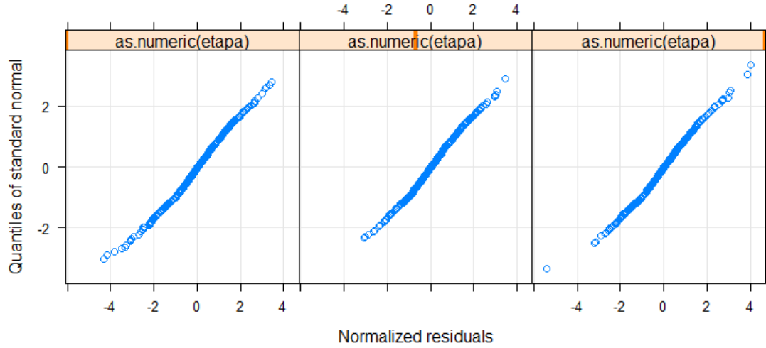
Figura 4.14: Escenario V - QQ plot: residuos normalizados.
